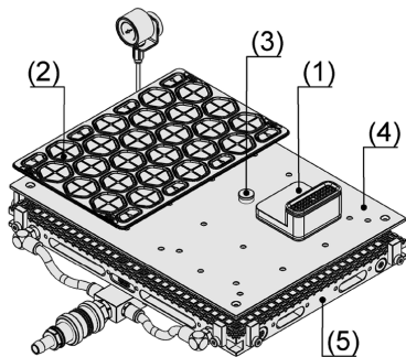
Конструкция системы Стальная плита Innospann ISST-MPL и блочная присоска ISBL
